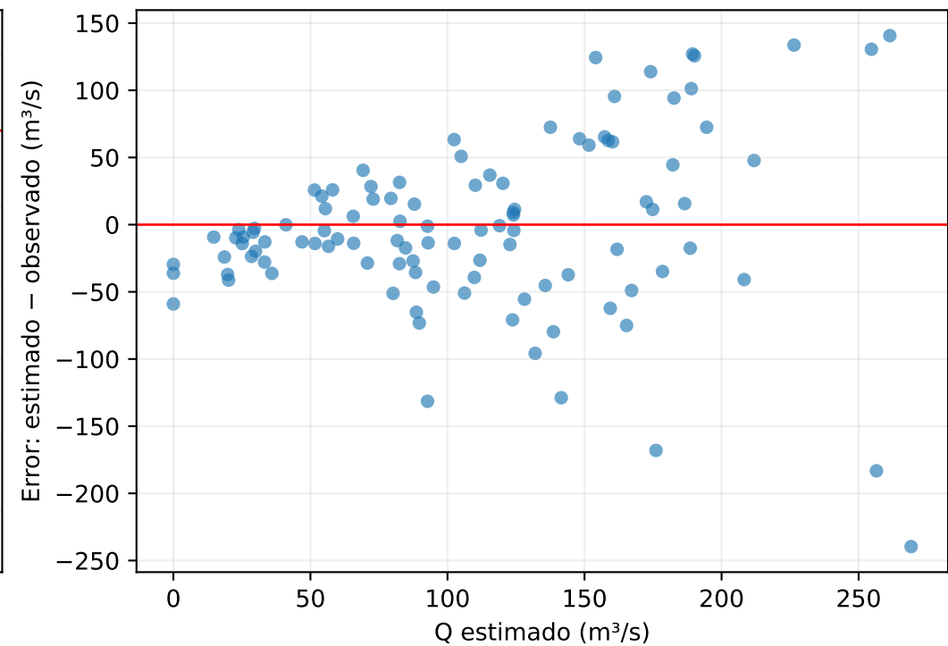
CHIRPS · errores de desarrollo
