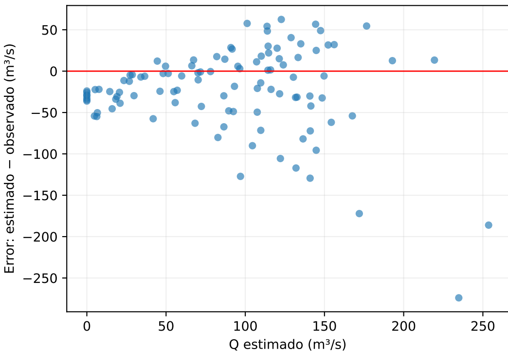
IMERG · errores de desarrollo
